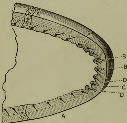
Fig. 87.—Lasting the Toe.
