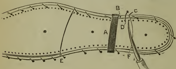
Fig. 90.—Sewing the Welt.
