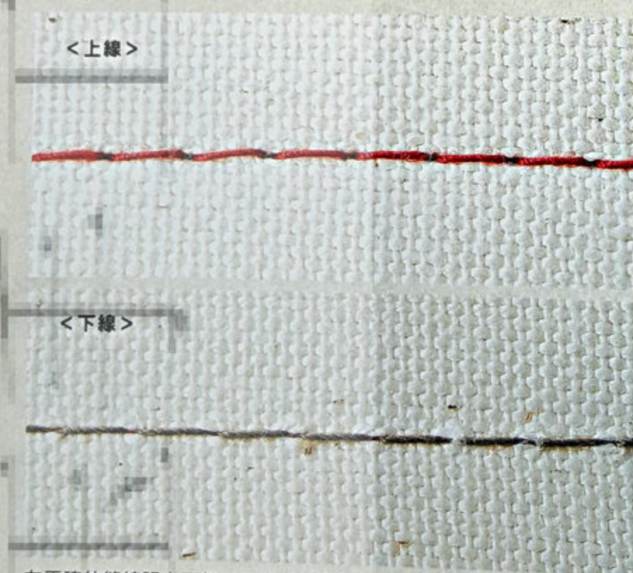
在正確的縫線張力下縫合後的正反面。不論從哪一面看都看不見相反面的縫線。
