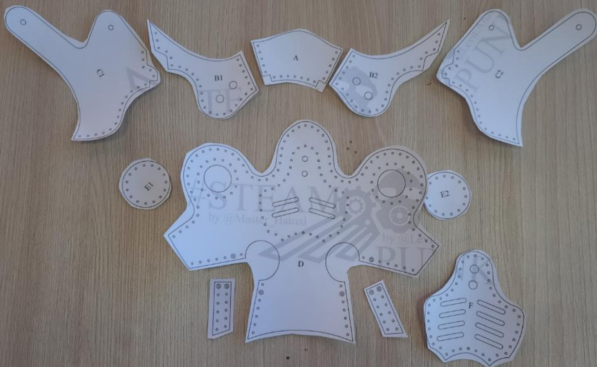
Step 4
