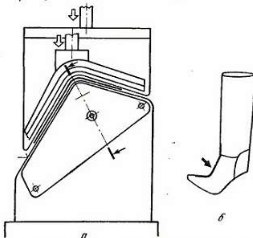
Рис. III.5. Схема формирующей пластины (а) и образец отформованного переда сапога (б)
