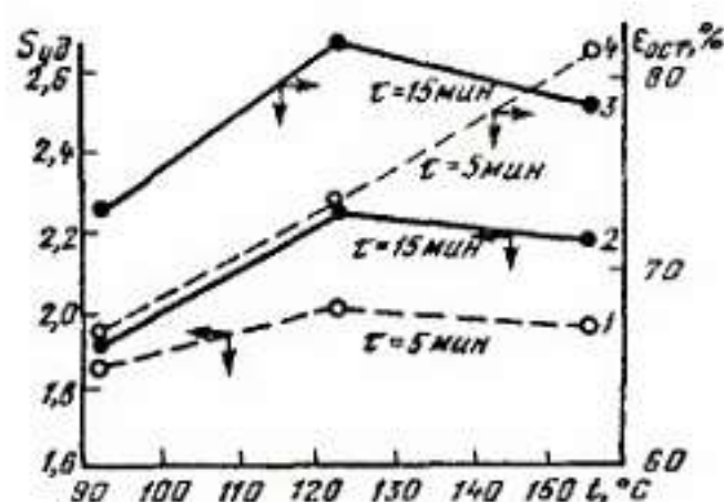
Рис. V.18. Изменение удельной поверхности пор (кривые 1 и 2) и остаточной деформации (кривые 3 и 4) винилскожи при тепловой фиксации формы обуви
