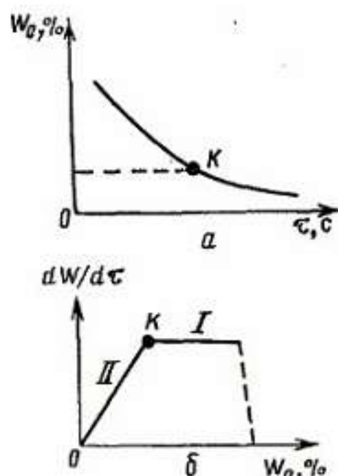
Рис. V.17. Кривые сушки (а) и скорости сушки (б)
