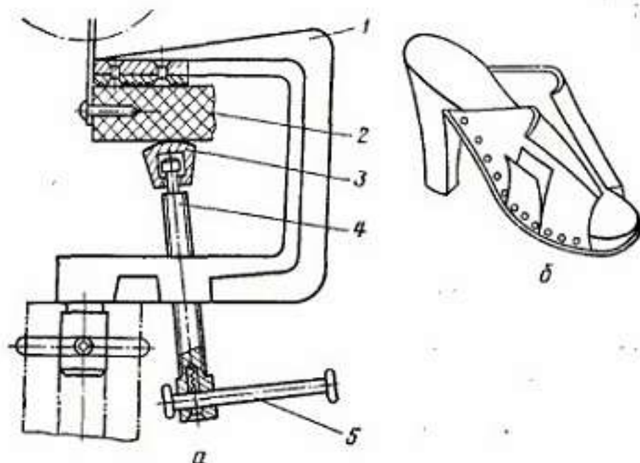
Рис. VIII.9. Приспособление к разрывной машине для определения прочности крепления подошвы гвоздебортного метода (а) и схема надрезания образца на заготовке верха обуви (б)
