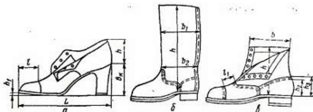
Рис. VIII.1. Определение линейных размеров обуви и ее деталей
