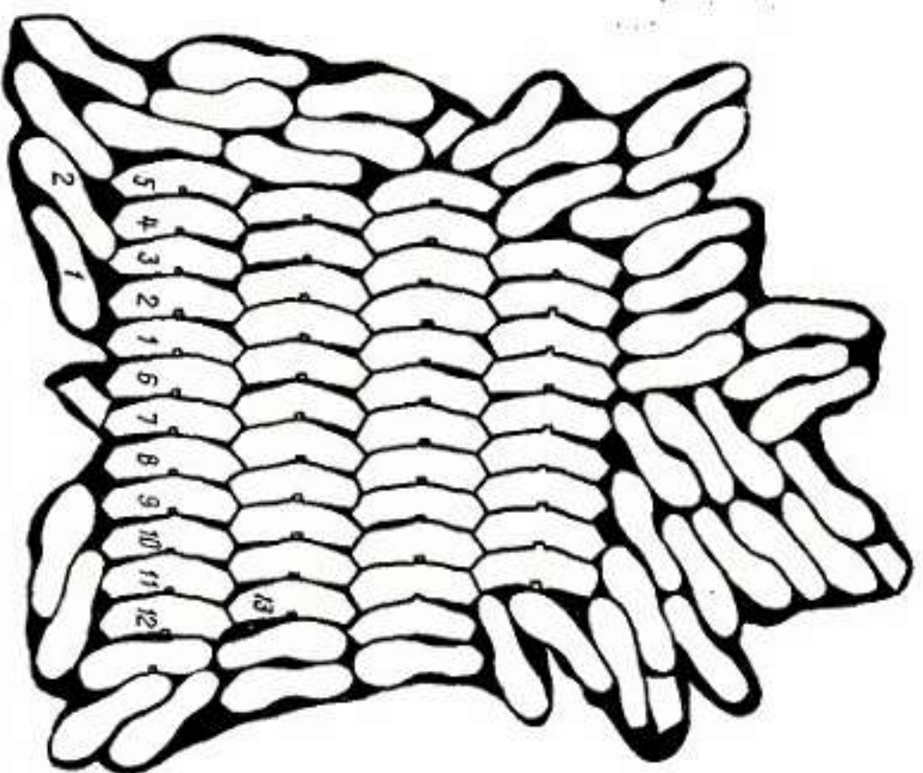
Рис. 1.16. Схема раскроя подкладочной кожи из выроста II сорта на детали подкладки женских сапожек (составлена В. И. Трошкиной)
