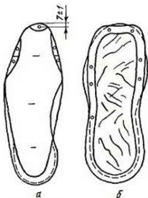
Рис. IV.15. Схема обтяжки заготовки верха обуви со свободной затяжной кромкой (а) и с пристроченным рантом (б)
