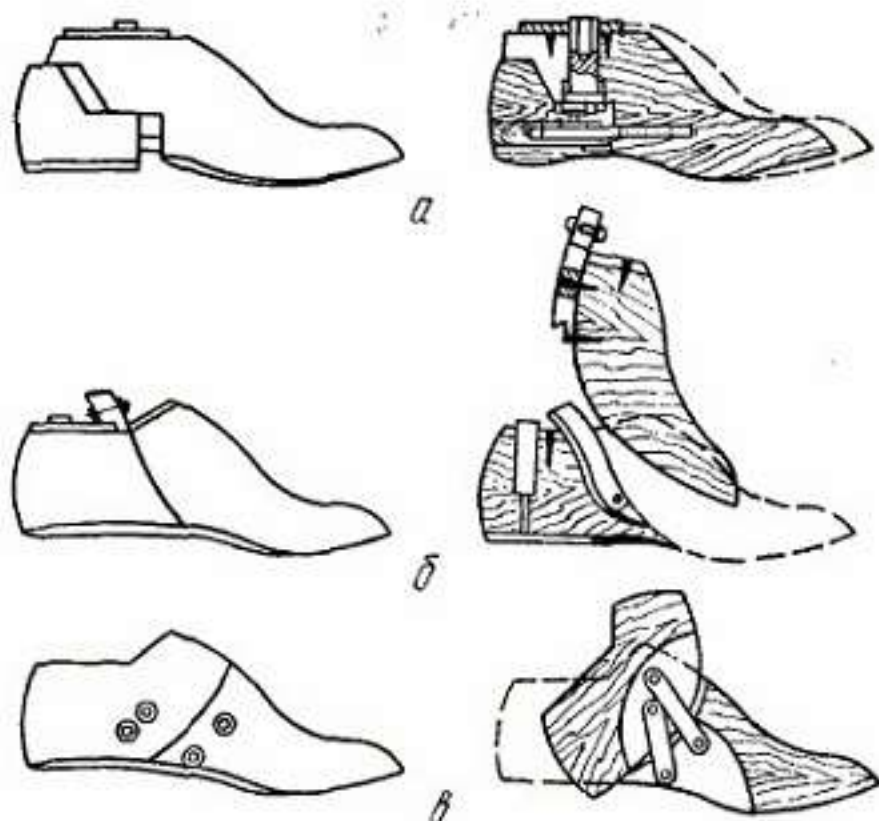
Рис. IV.10. Схемы раздвижных колодок
