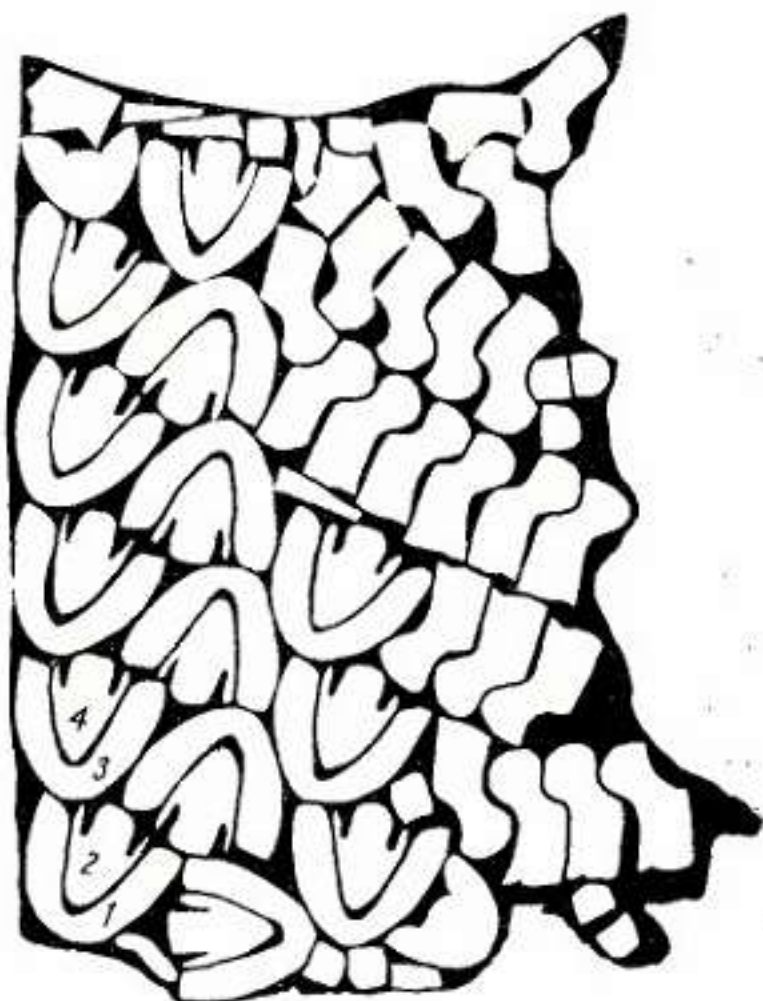
Рис. 1.6. Схема раскроя полукожи без воротка II сорта из шкур крупного рогатого скота на детали мужских модельных полуботинок в комбинации с деталями дошковых II подгруппы ботинок (составлена Л. И. Кахныч)
