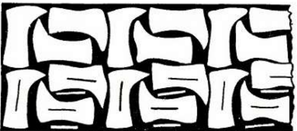
Рис. 1.26. Схема раскрой искусственной кожи на детали верха женских сапожек (составлена Московским ТПОО «Заря»)
