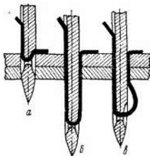
Рис. III.9. Схема образования петли
