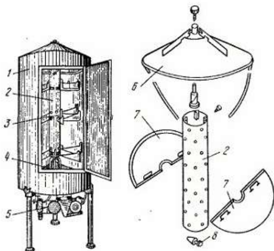
Рис. V.6. Схема установки для увлажнения водяным туманом:
