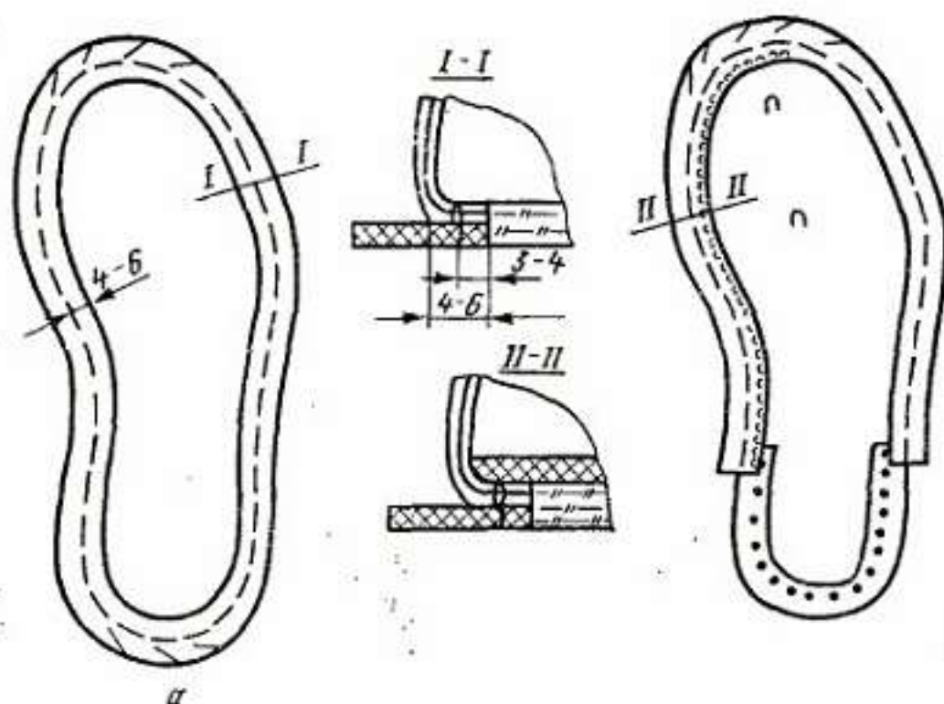
Рис. VI.20. Схемы протирания следа обуви, изготовленной методами «ларко-1» (а) и «ларко-2» (б)
