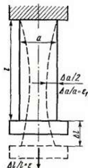
Рис. IV.3. Схема растяжения сетчатых материалов
