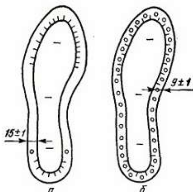
Рис. IV.19. Схемы затяжки геленочной части заготовки верха
