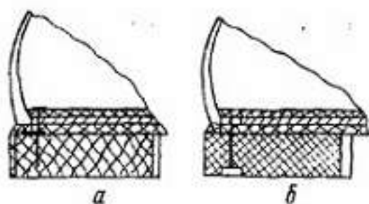
Рис. VI.24. Схемы прикрепления низких каблучков кожаного изнутри (а) и резинового снаружи (б)
