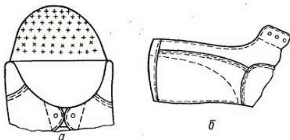
Рис. IV.13. Схемы вклеивания подноски (а) и задника (б)
