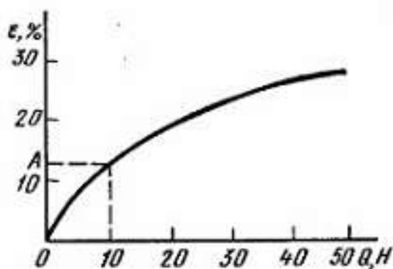
Рис. IV.2. Кривая растяжения сетчатого материала
