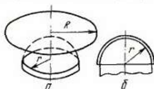
Рис. IV.4. Схема формования круга из кожи на полусфере
