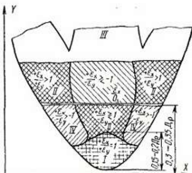
Рис. IV.8. Характер сложного напряженного состояния отформованной союзки
