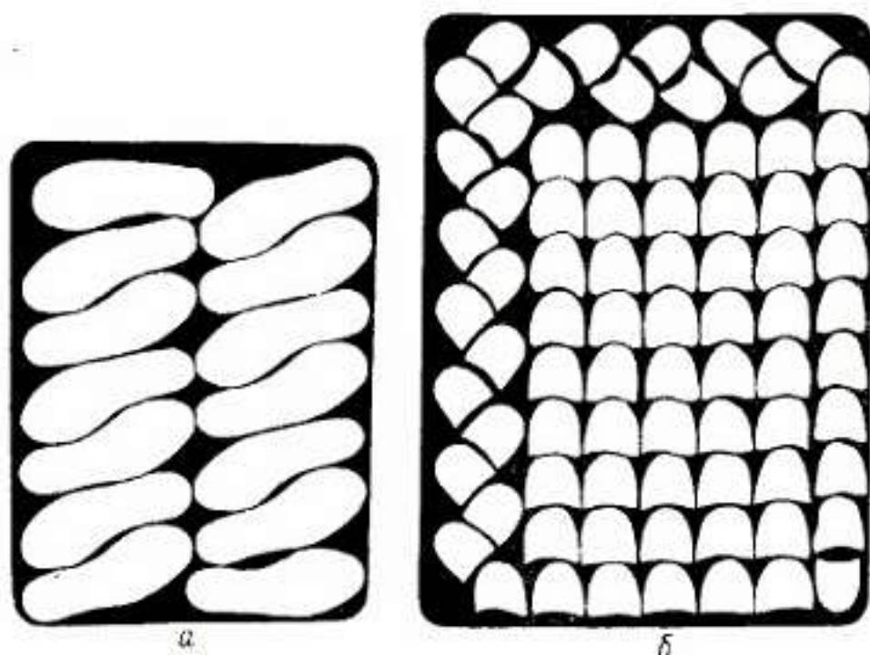
Рис. 1.33. Схемы разруба резиновых пластин: а — на мужские подошвы (составлена В. И. Терешко); б — ва каблук для школьных туфель (составлена В. И. Терешко)
