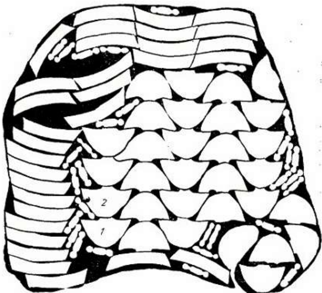
Рис. 1.11. Схема раскроя обувного свилка I сорта на детали школьных летних туфель (составлена Н. И. Сокальчук)
