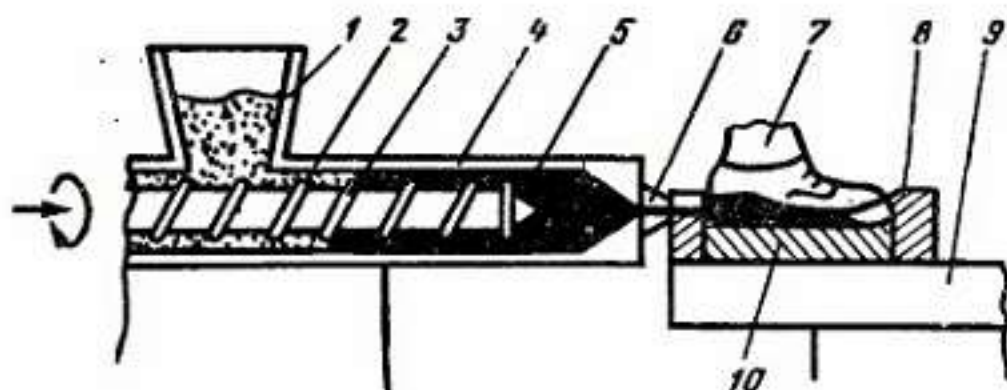
Рис. VI.7. Схема литья низа обуви:
