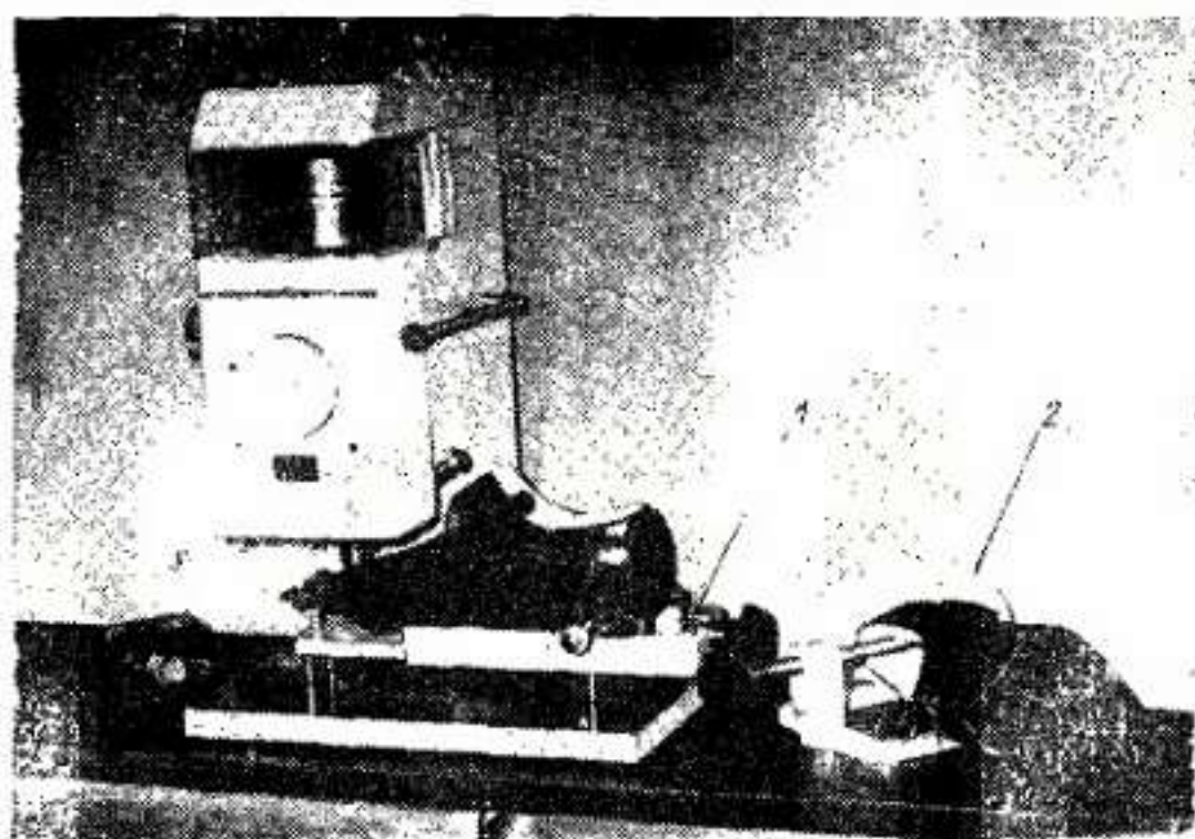
Рис. VIII.12. Прибор ЖНЗО-2 для определения обшей и остаточной деформации подноски и задника обуви с приспособлениями 1 и 2 для испытания подноски и задника
