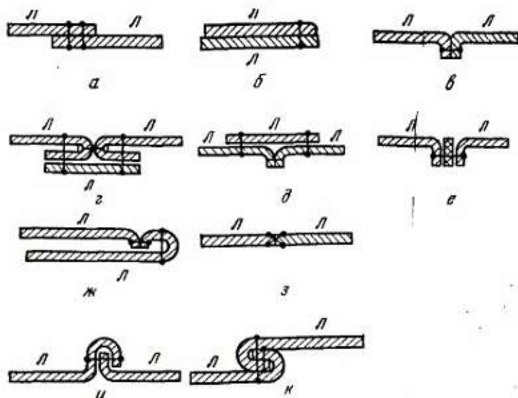
Рис. III.16. Швы для скрепления деталей верха обуви
