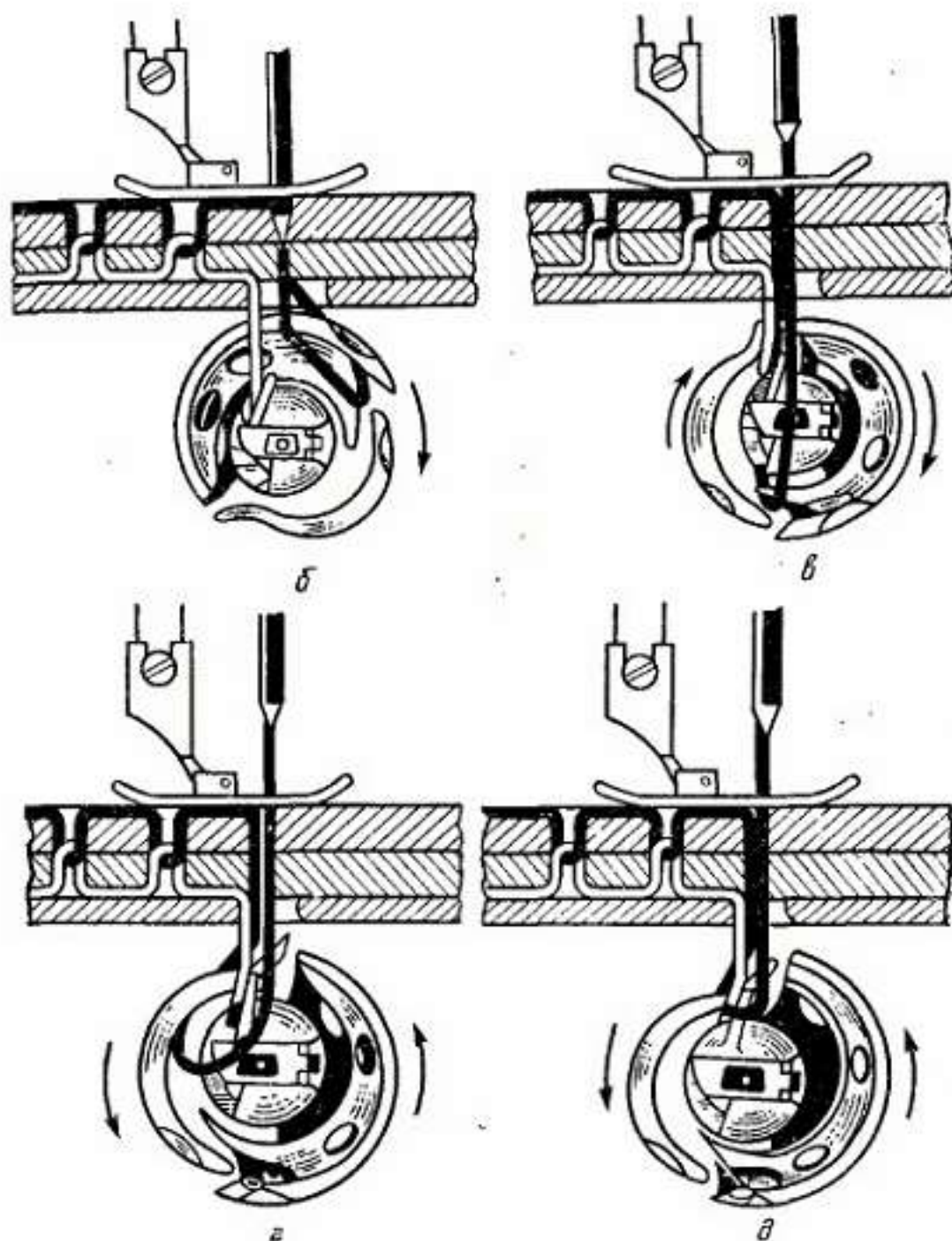
Рис. III.10. Процесс образования двухниточного стежка внутреннего переплетения на швейной машине с качающимся челноком
