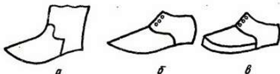
IV.1. Конструкция передней части заготовки верха: а — плоская; б — полуплоская; в — пространственная
