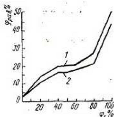
Рис. V.1. Зависимость влажности кож хромового (1) и хромтанидного (2) дубления от относительной влажности воздуха.
