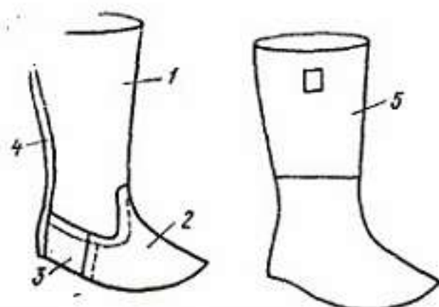
Рис. 111.32. Детали верха сапог с голенищами из юфти:
