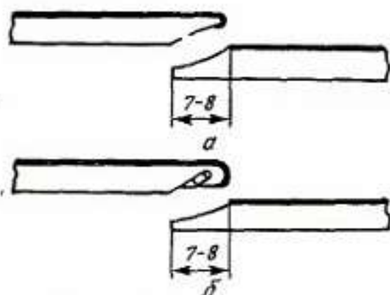
Рис. III.6. Виды обработки краев деталей верха при склеивании клеевым методом
