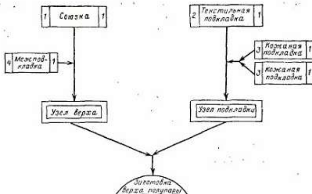
Рис. 111.25. Схема сборки заготовки перха туфель-лодочек с круговой союзкой
