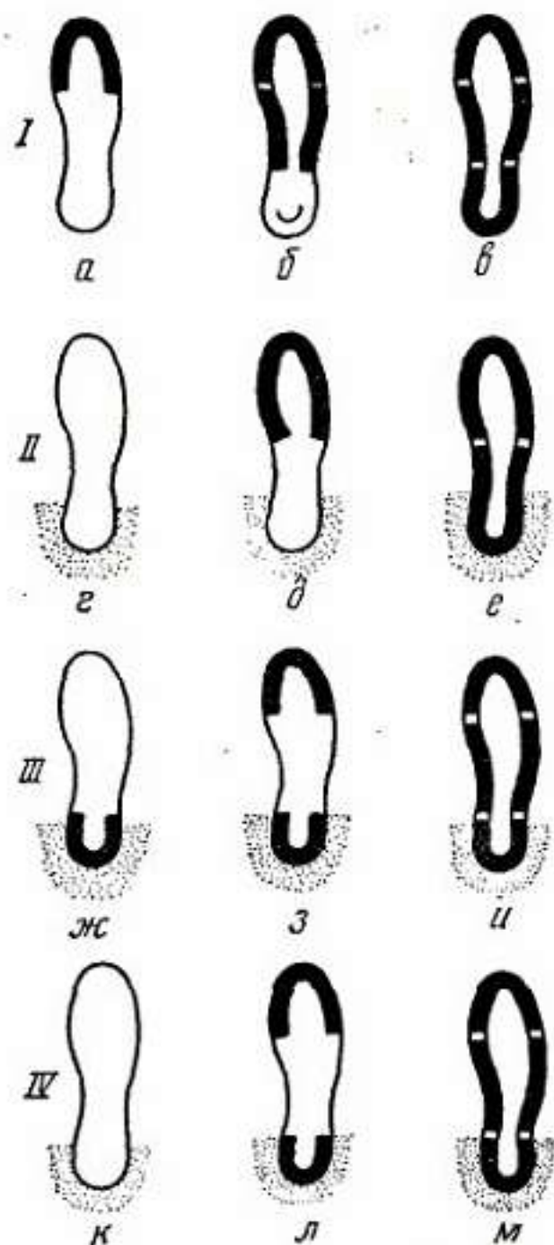
Рис. IV.9. Варианты формирования заготовок верха обуви обтяжно-затяжным методом
