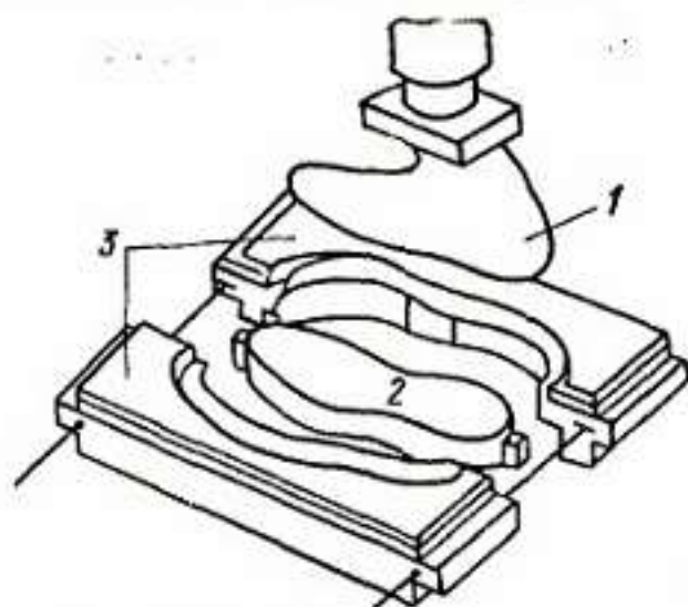
Рис. VI.4. Схема пресс-формы
