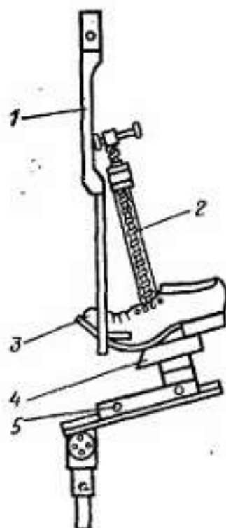
Рис. VIII.15. Прибор для определения гибкости обуви
