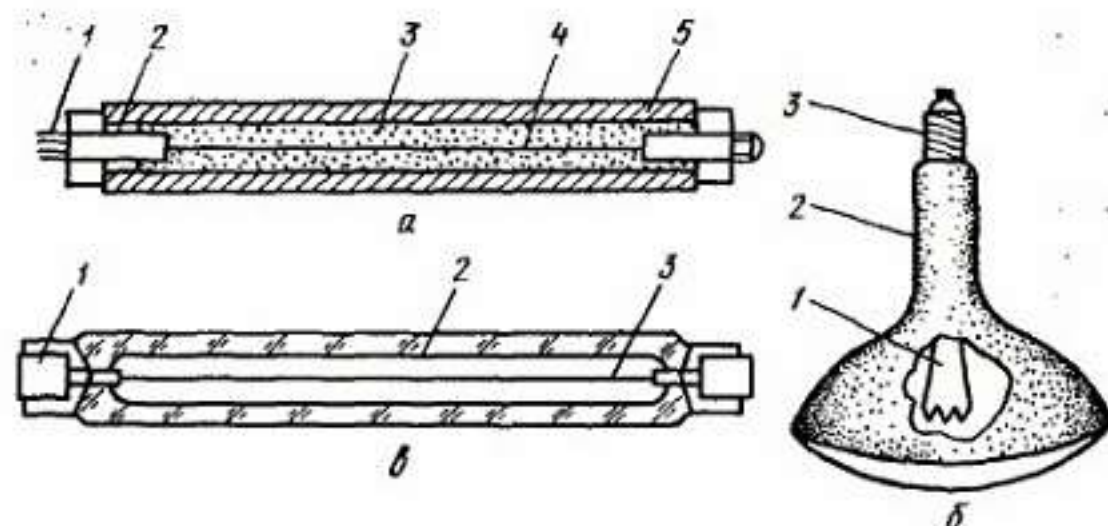
Рис. V.11. Схема инфракрасных излучателей:
