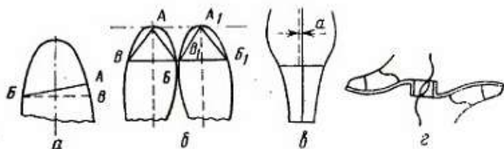
Рис. VIII.2. Определение перекосов, симметричности расположения деталей
