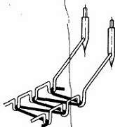
Рис. III.15. Трехниточный цепной стежок наружного переплетения
