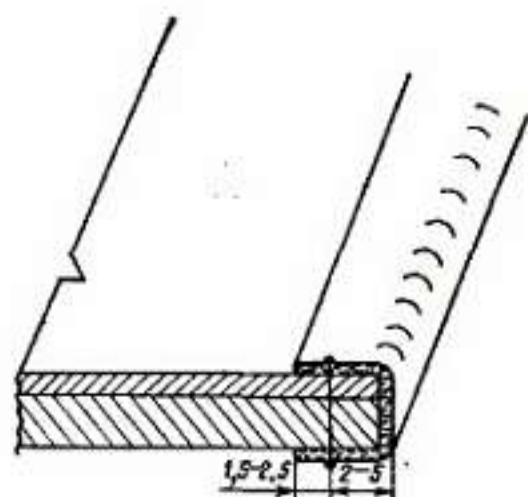
Рис. III.2. Окантовывание края детали
