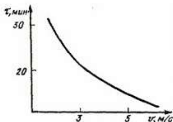
Рис. V.8. Зависимость времени сушки от скорости воздуха
