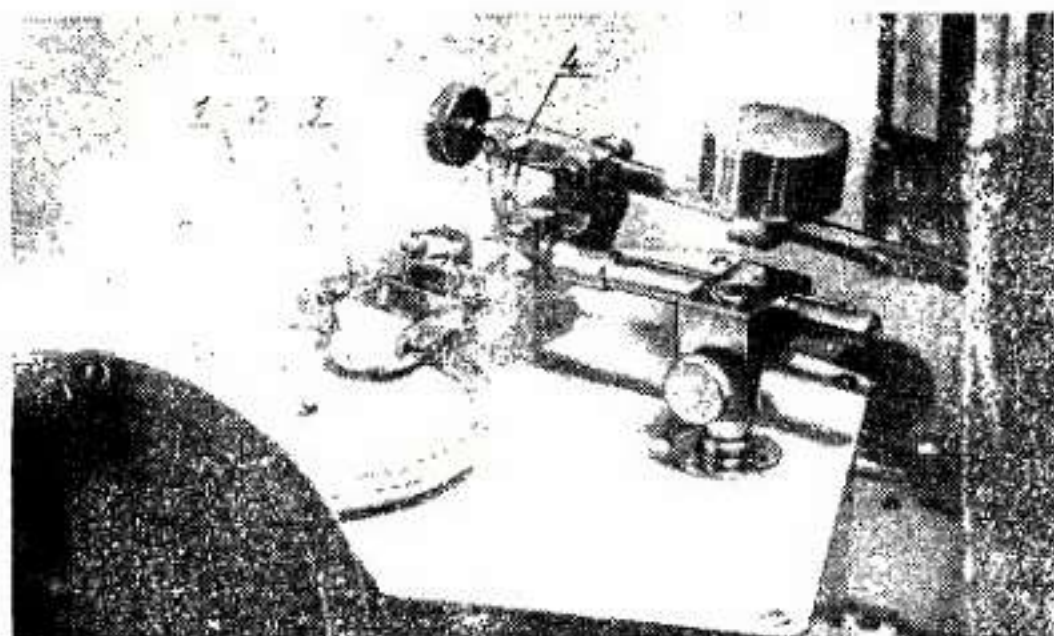
Рис. VIII.20. Прибор для измерения величины и знака электрических зарядов на образцах материалов и систем материалов: 1 — диск для закрепления второго компонента пары трения; 2 — головка для закрепления пластины с наклеенным испытуемым образцом; 3 — датчик измерителя; 4 — механизм нагружения образца.
