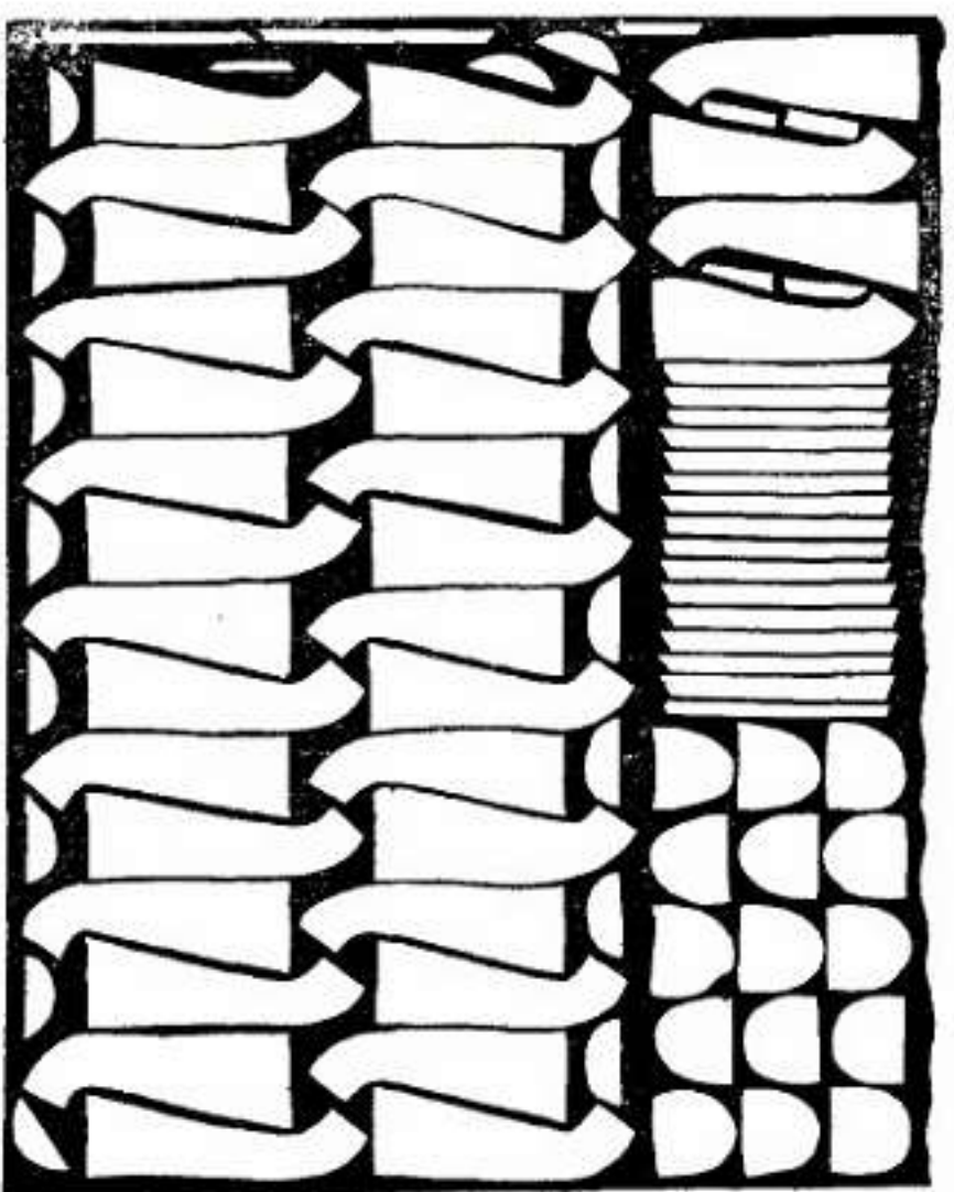
Рис. 1.27. Схема раскрой синтетической кожи на детали верха мальчиковых летних туфель (составлена Г. А. Назаровой)
