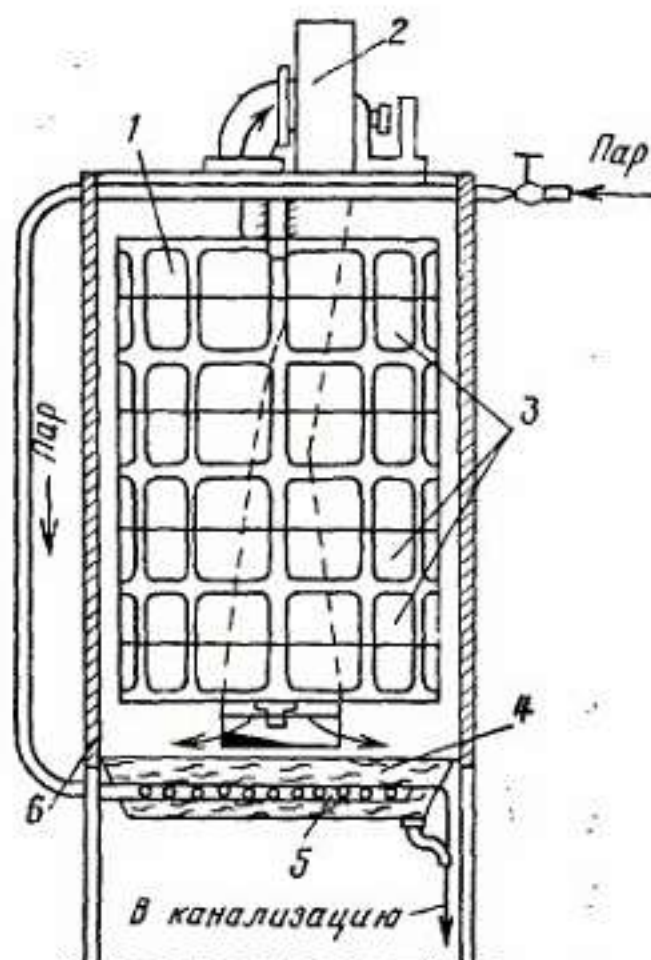
Рис. V.5. Схема установки для увлажнения деталей низа обуви
