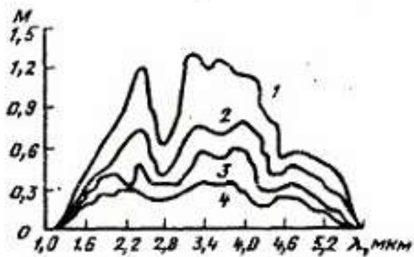
Рис. V.13. Кривые относительного спектрального распределения энергии ТЭНов при напряжении, В: 1 — 220; 2 — 200; 3 — 180; 4 — 160
