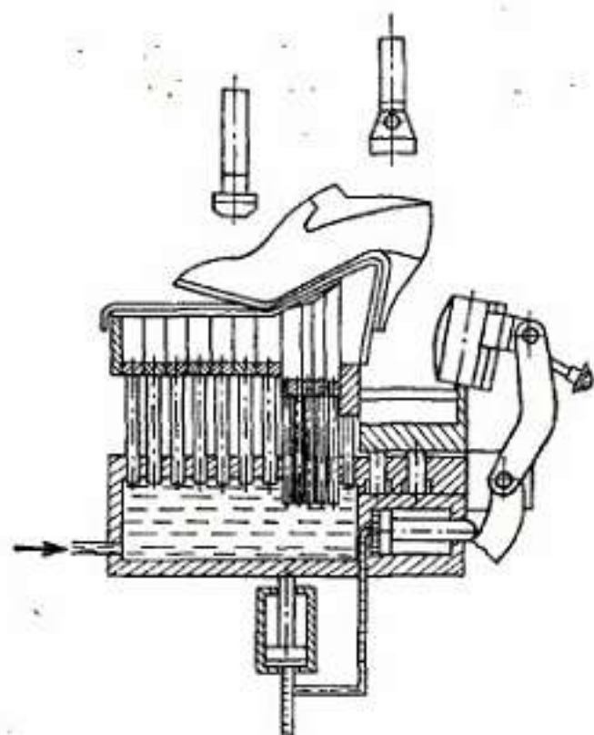
Рис. VI.2. Схема универсальной пресс-секции с резиновыми клавишными прижимами
