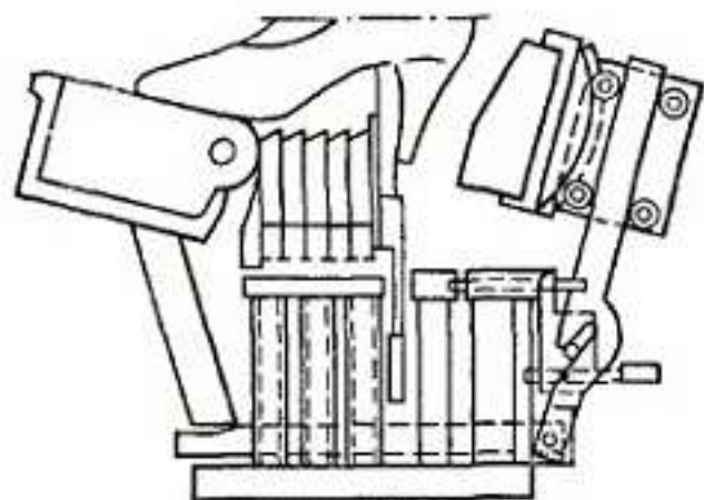
Рис. VI.3. Схема универсальной пресс-секции пресса С фирмы УСМ
