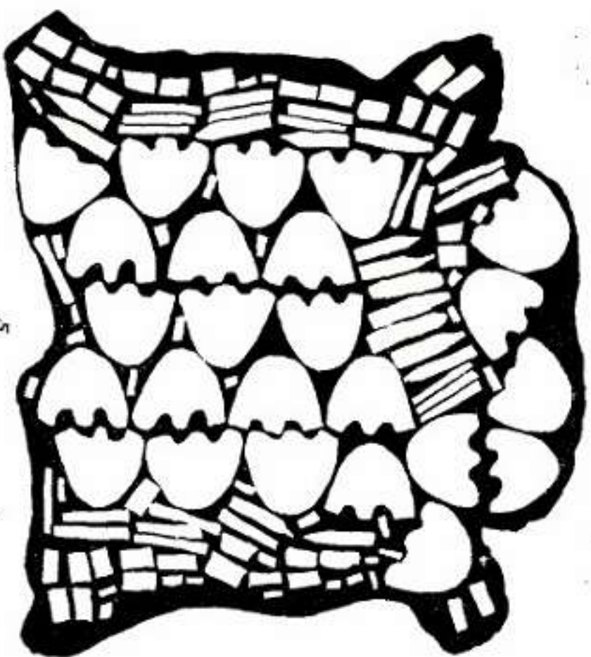
Рис. 1,15. Схемы раскром юфти на детали сапог и полусапог (а) при соотношении нар 6 : 2,5, детали сапог с кир- совыми голенищами (б) (составлены Е. Е. Патрикеевой)
