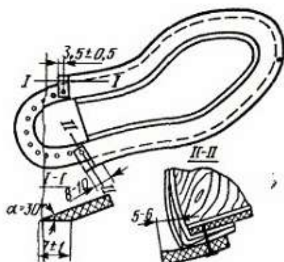
Рис. VI.13. Схема спускания и закрепления концов ранта
