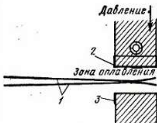
Рис. III.7. Схема контактно-тепловой сварки
