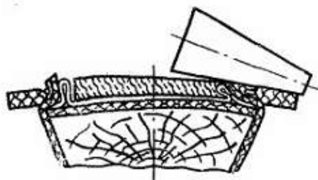
Рис. VI.12. Схема прессования узла рант—губа стельки
