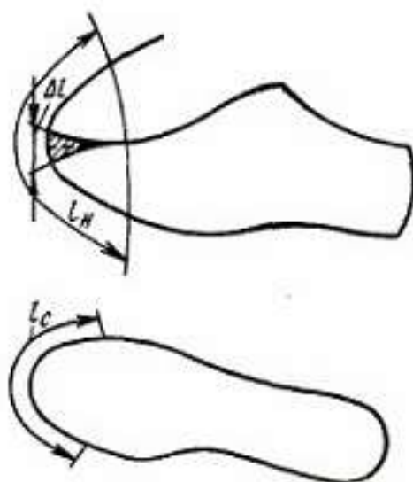
Рис. IV.5. Схема определения коэффициента посадки носка
