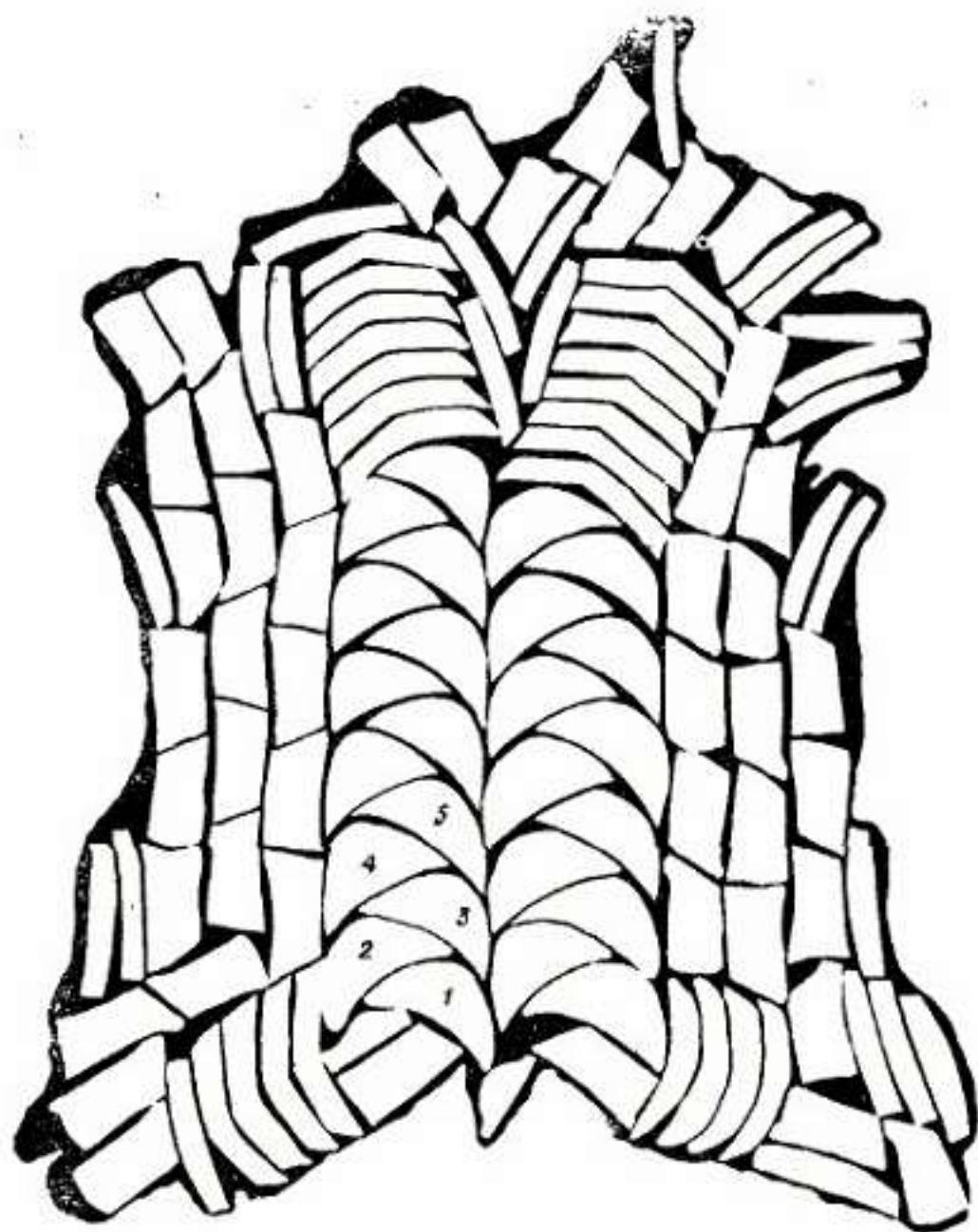
Рис. 1.5. Схема раскроя лаковой кожи 1 сорта из шкур крупного рогатого скота на детали женских модельных туфель и обтяжку каблука (составлена В. И. Трошкиной)
