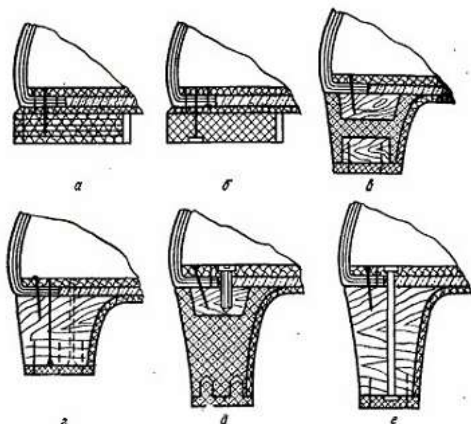
Рис. VI.23. Схемы способов прикрепления каблучков: а — низкого кожаного гвоздями изнутри; б — низкого резино- ного формованного клеем и гвоздями снаружи; в — среднего пластмассового клеем и гвоздями изнутри; г — среднего дере- вянного клеем, насадочными гвоздями снаружи и гвоздями изну- три; д — высокого пластмассового клеем, шурупом и гвоздями изнутри; е — высокого деревянного клеем, ступкой и гвоздями изнутри
