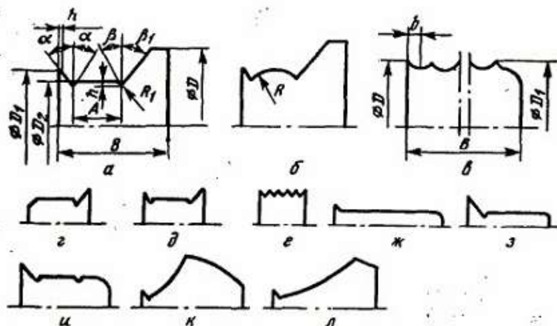
Рис. VII.2. Формы полок зубьев прямой (а) и выпуклой (б) для обработки подошв, фигурной (в) для обработки уреза пористых подошв, для обработки набоек (г, д, е), для обработки каблучков (ж, з), для подправки уреза на участке перехода от геленочной части к каблучной и обработки подошвы с утолщенной пяточной частью (и), геленочных фрез (к, л)
