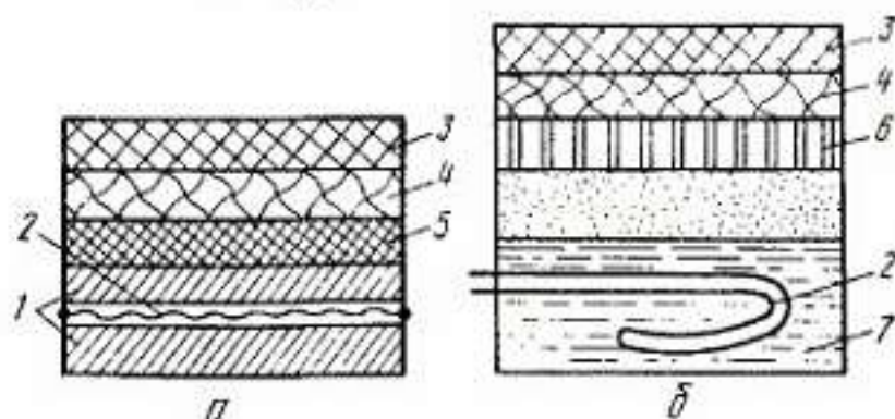
Рис. V.3. Схемы установок для контактного увлажнения материалов
