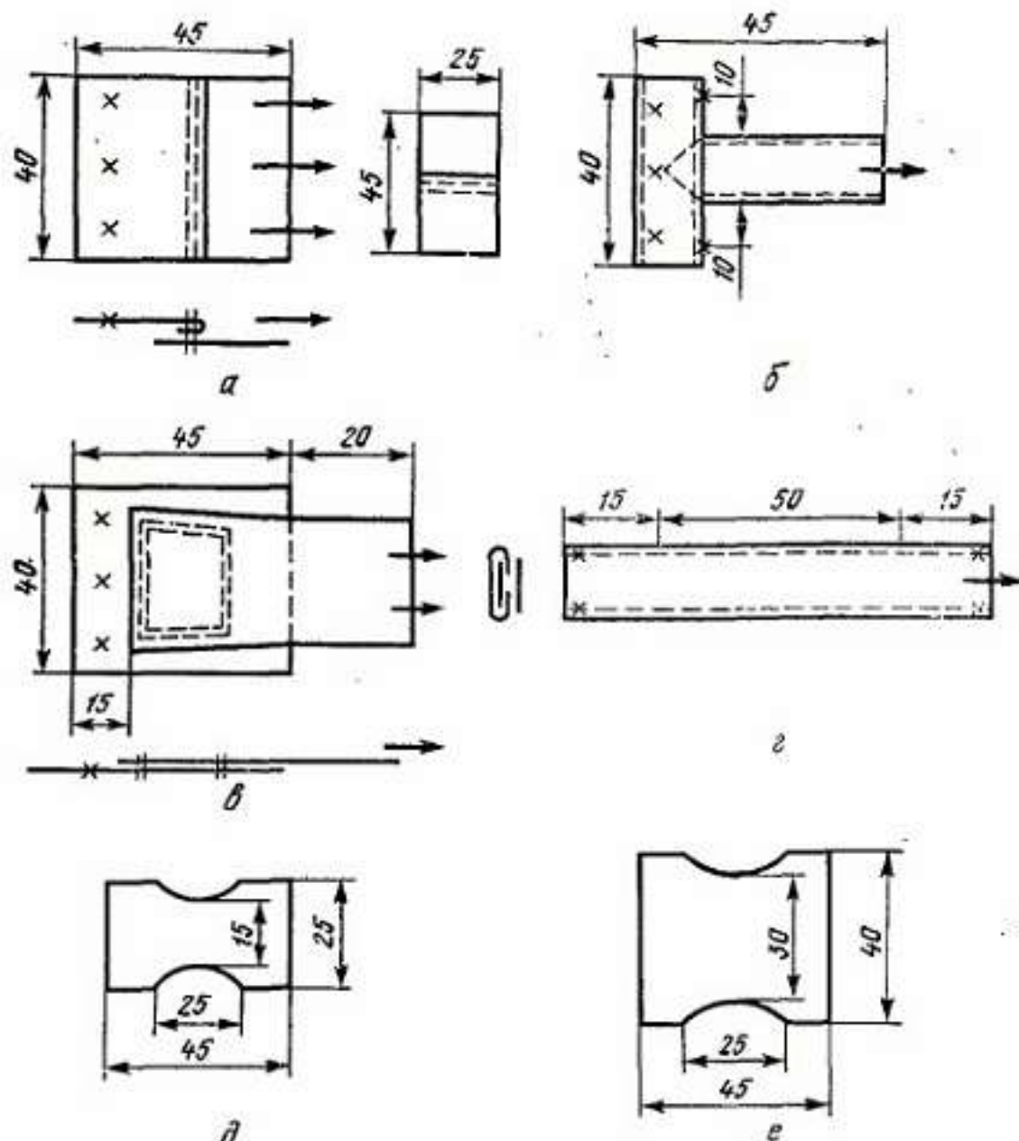
Рис. VIII.5. Форма и размеры простроченных образцов для определения прочности швов заготовок верха обуви (а), ремешков (б), продольных ремней (в) и ремешков (г), испытывающих наибольшие напряжения, и простроченных образцов для задники (д), союзки и берцов (е)
