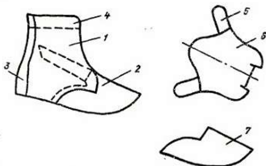
Рис. III.36. Детали полусаног с верхом из юфти.
