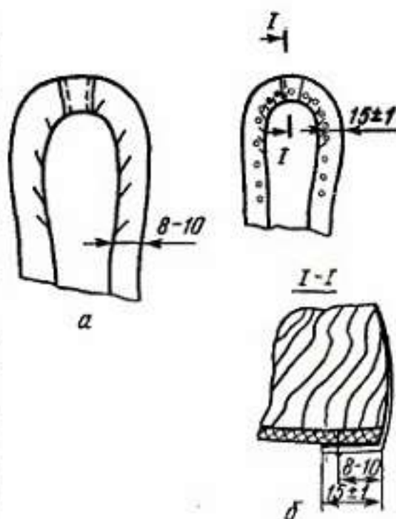
Рис. IV.17. Схемы затяжки пяточной части заготовки верха обуви
