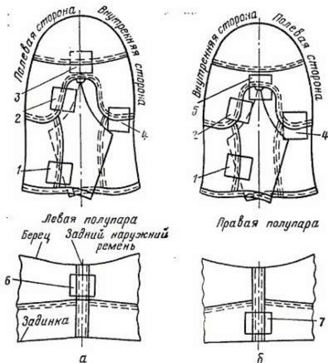
Рис. VIII.3. Расположение на заготовках верха полусапог, ботинок, полуботинок и туфель образцов для определения прочности швов левой (а) и правой (б) полупар:
