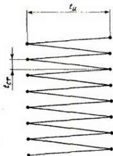
Рис. III.12. Параметры зигзагообразной строчки
